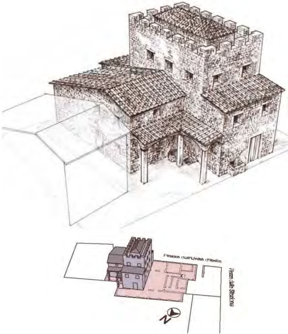
Figura 60: Ricostruzione grafica del complesso nella Fase 11 EST, con la loggia angolare e l'abitazione ottenuta dalla turris e dal cortile antiporta ormai coperto (Simone Boni per Inklink)
