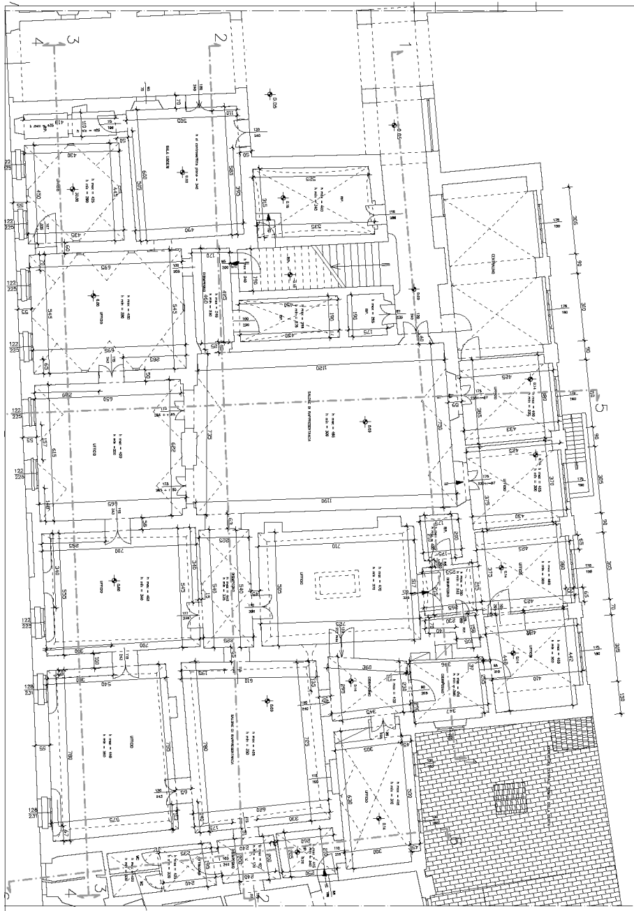
Figura 1: Pianta complessiva del piano terra di Palazzo Cerretani prima dei lavori
