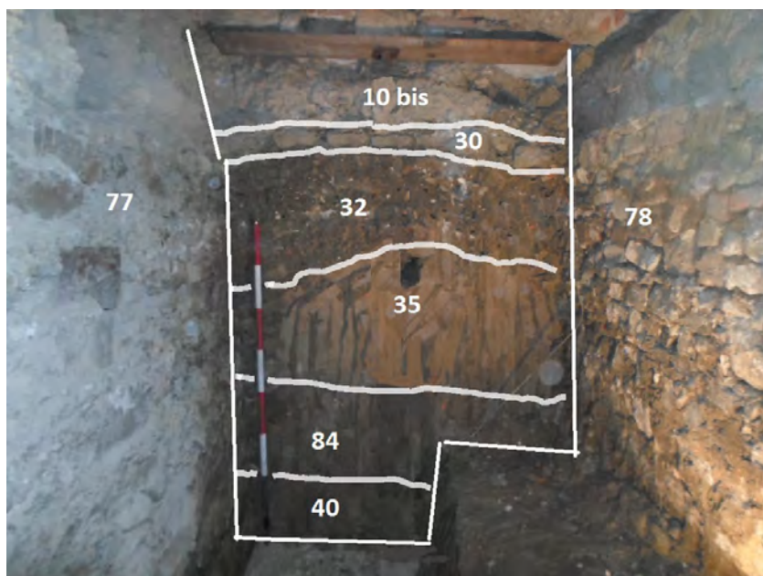
Figura 37: L'indagine dello spazio indisturbato sotto il vano PT 27 con evidenziate le UUS
